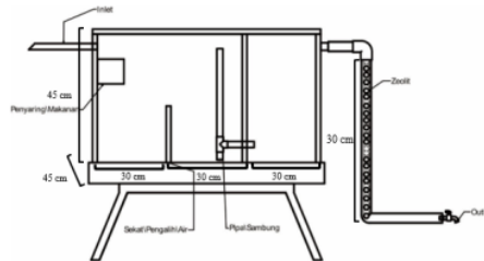
Gambar 1. Desain Alat Penelitian
