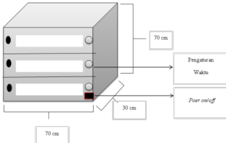
Gambar 1 Tampak Depan Lemari
